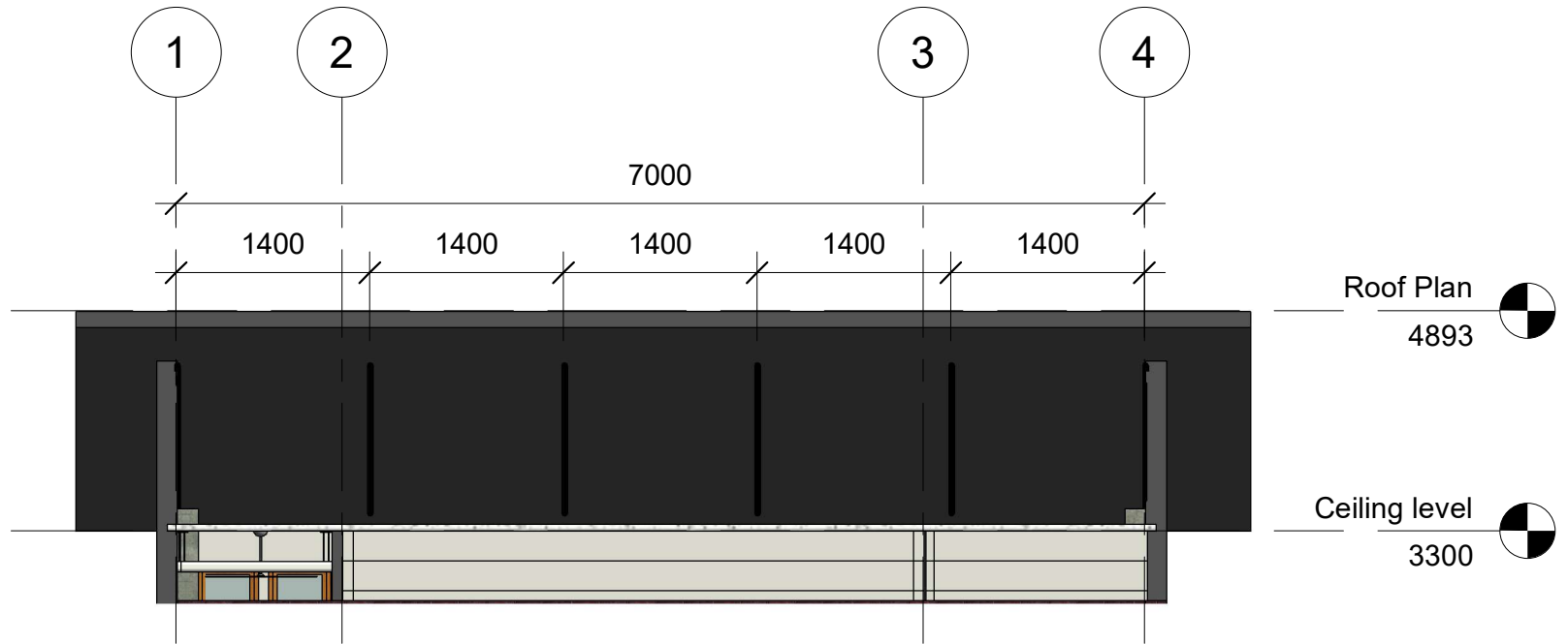
1 Roof Section A-A 1 : 50
