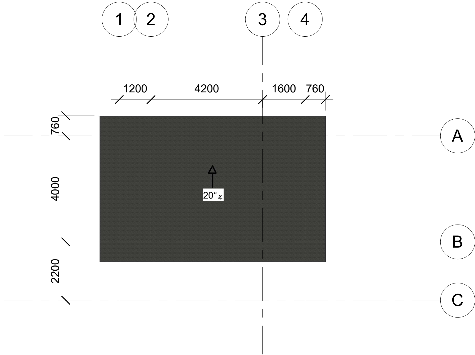
1 Roof Plan 1 : 100
