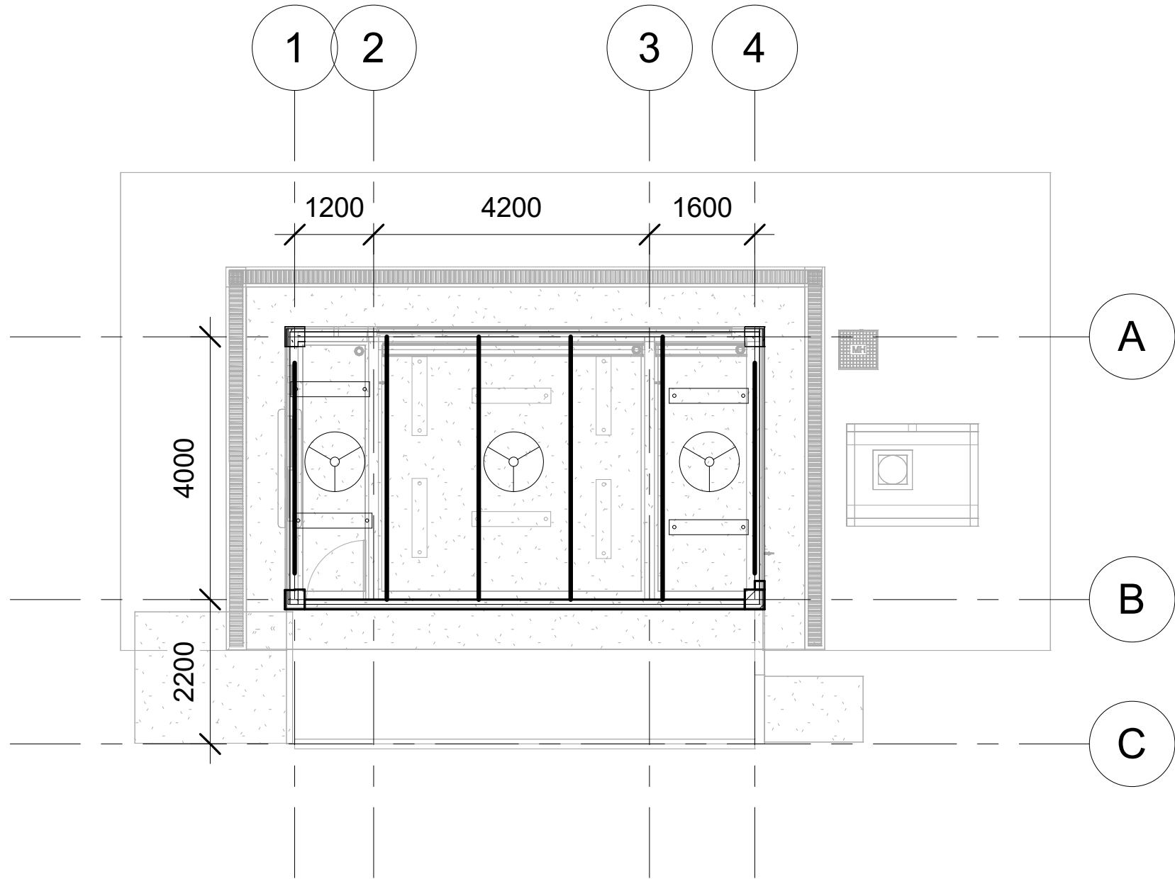
1 Electrical Point Plan 1 : 100
